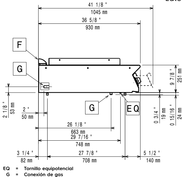
Planta
